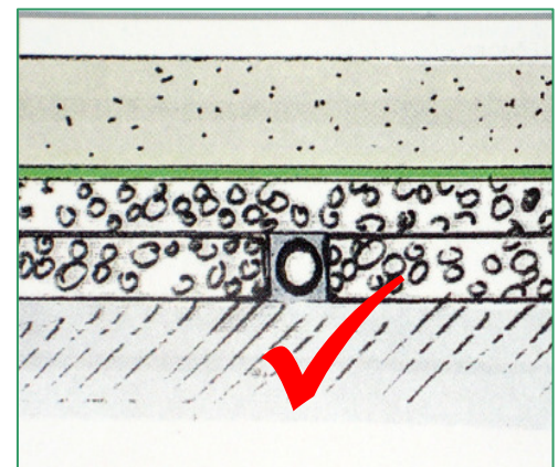
Beispiel einer korrekten Verlegung der Zuleitung zu Heizelementen
